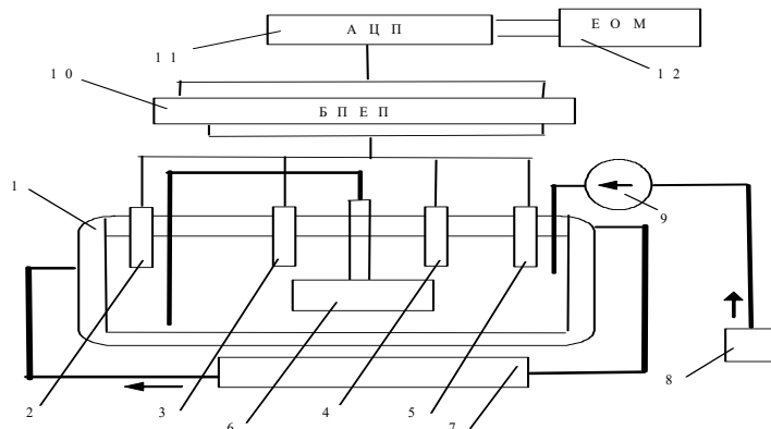
Рис. 1. Блок-схема установки для дослідження ефективності дії інгібіторів відкладень: 1 – термостатована комірка, 2 – електрод порівняння, 3 – pH -електрод, 4 – pCa -електрод, 5 – температурний давач, 6 – насос перемішування, 7 – термостат, 8 – ємність для NaOH , 9 – перистальтичний насос, 10 – БПЕП, 11 – плата АЦП, 12 – ЕОМ
