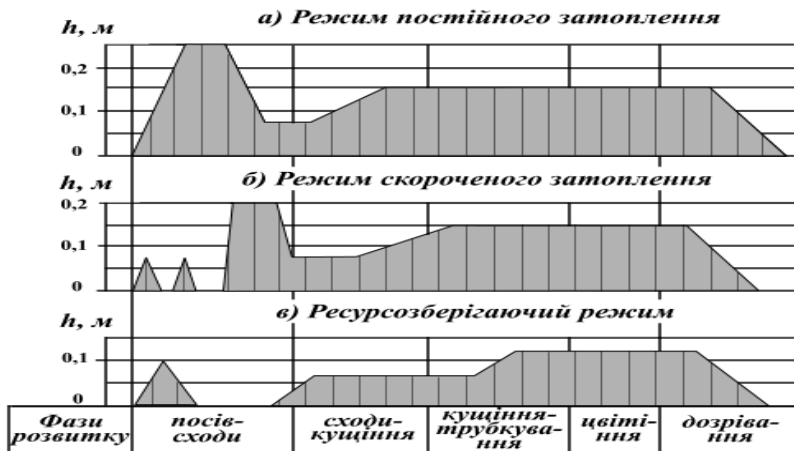
Рис. 1. Схема реалізації основних режимів зрошення при поверхневому затопленні за фазами розвитку рослини рису
