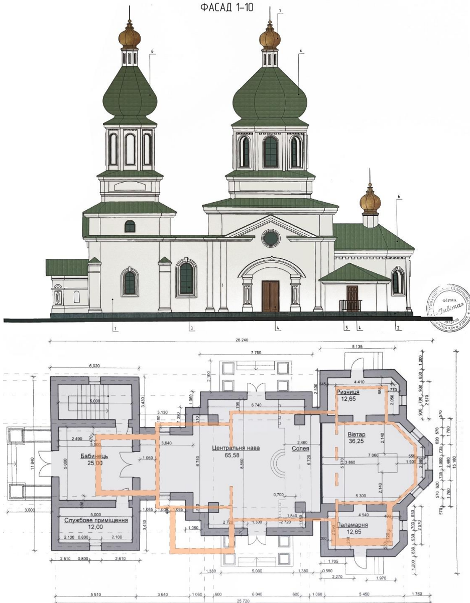
Рис. 5. Проектні креслення нового Свято-Георгіївського храму в с. Колоденка, надані настоятелем Петром Велігурським: південний фасад і план першого поверху з нанесеними стінами існуючої дерев'яної церкви (виділено червоним кольором). Джерело: опрацювання П. Фенюком.
