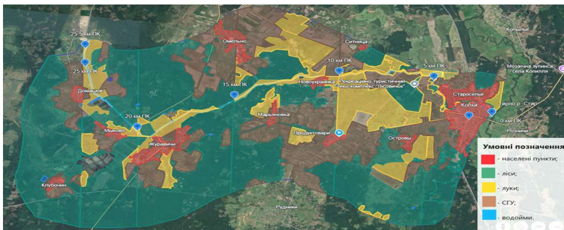
Рис. 2. ПТК басейну річки Рудка станом на 2021 рік
