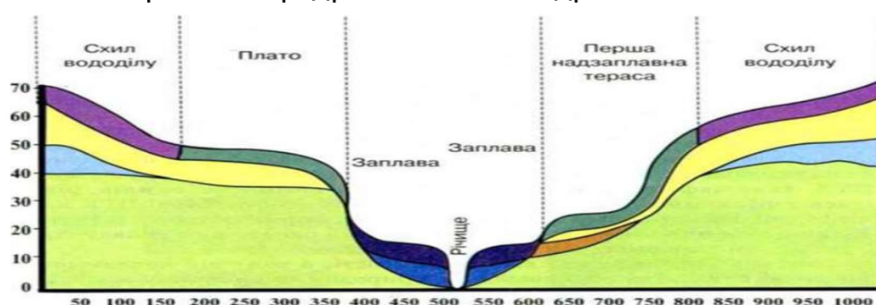
Рис. 1. Схема ПТК річкової долини
