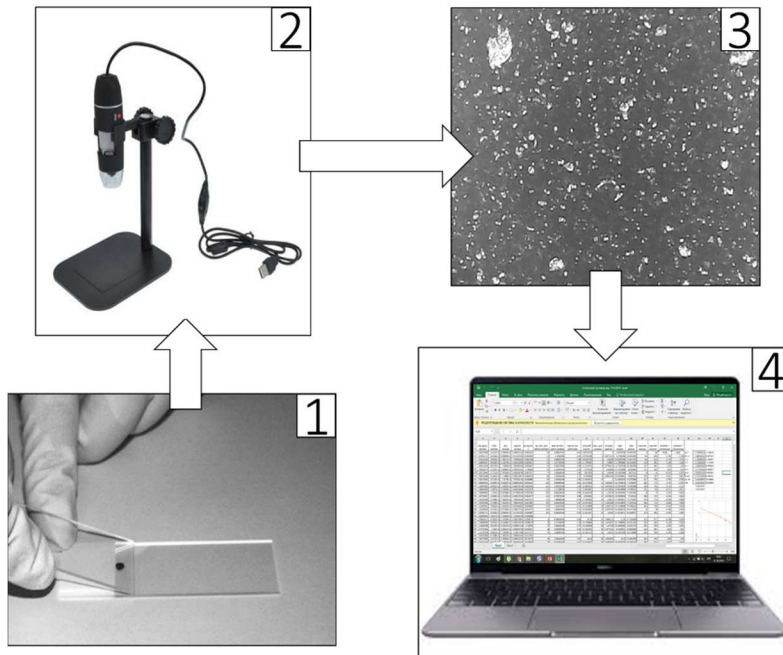
Рис.1. Визначення дисперсного складу стічних вод за допомогою цифрового USB-мікроскопу з подальшим застосуванням системи аналізу оптичних зображень на комп'ютері:
