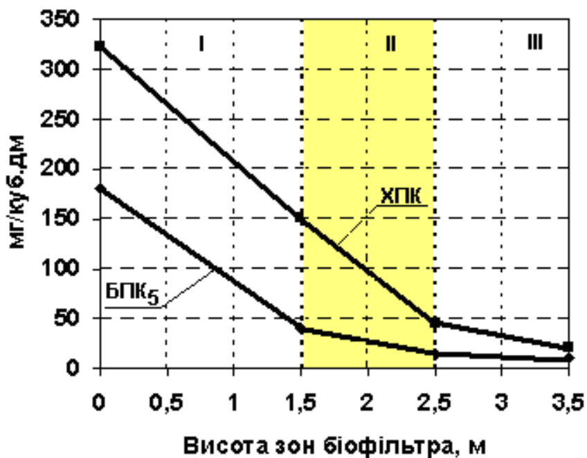
Рис. 2. Динаміка зміни концентрації органічних забруднень стоків у кожній зоні біофільтра за BPK 5 і ХПК
