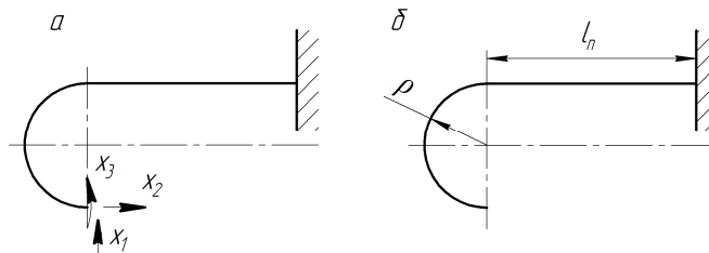
Рис. 3. Еквівалентна (а) і основна (б) системи пружної частини шпонки
