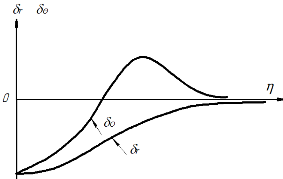
Рис. 1. Епюри напружень \sigma_r та \sigma_\theta (плоска задача)
