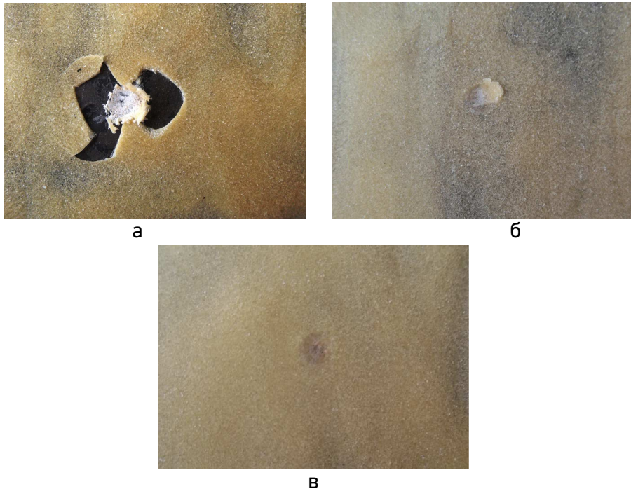
Рис. 4. Загальний вигляд поверхні двошарових покриттів оброблених ультразвуком після досліджень на ударну міцність при використанні в якості ґрунтового шару: а – епоксиолімеру; б – епоксикомпозиту з порошком цирконію; в – епоксикомпозиту з карбонільним залізом
