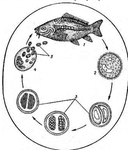
Рисунок. Цикл розвитку Ichtyophthirius multifiliis : 1 – риба – дефінітивний живитель; 2 – зрілий трофозоїт; 3 – поділ паразита; 4 – циста; 5 – вихід «бродяжок»
